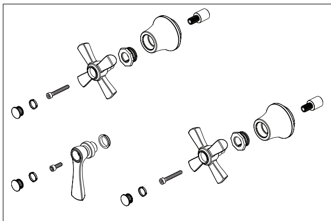
RP93875▲ Handle Kit Juego de piezas para las manijas Trousse de manettes
