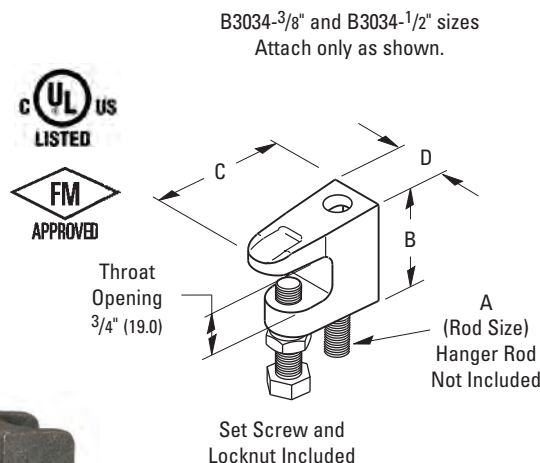
B3034-3/8 Shown
