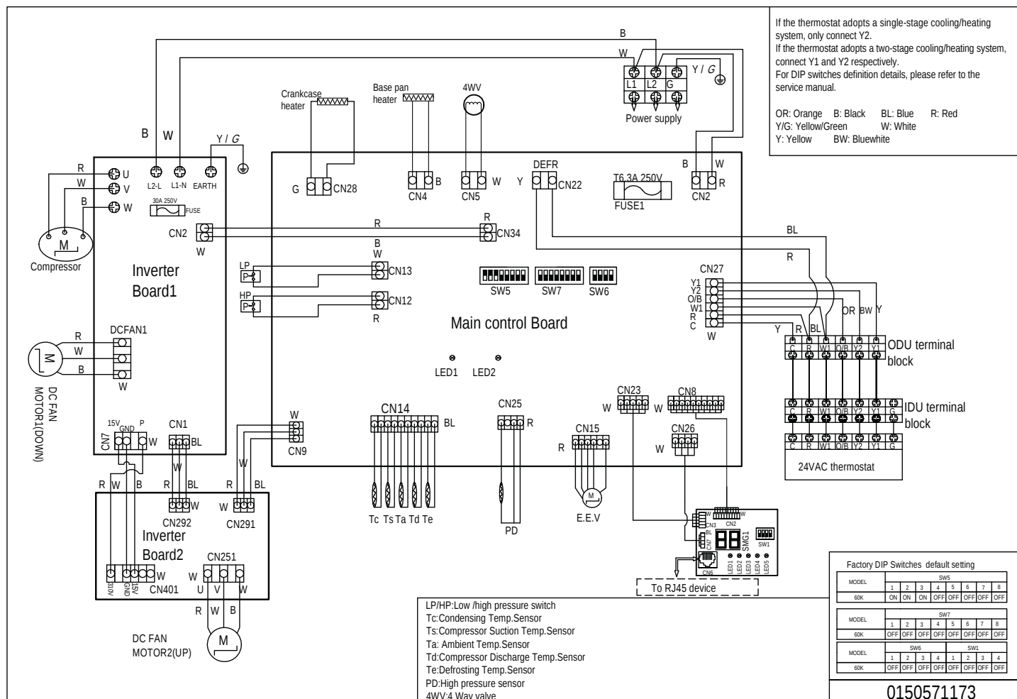
Figure 22. Schéma de câblage 60K.
