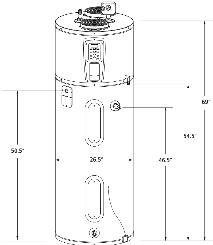
HPAX-80 dimensions
