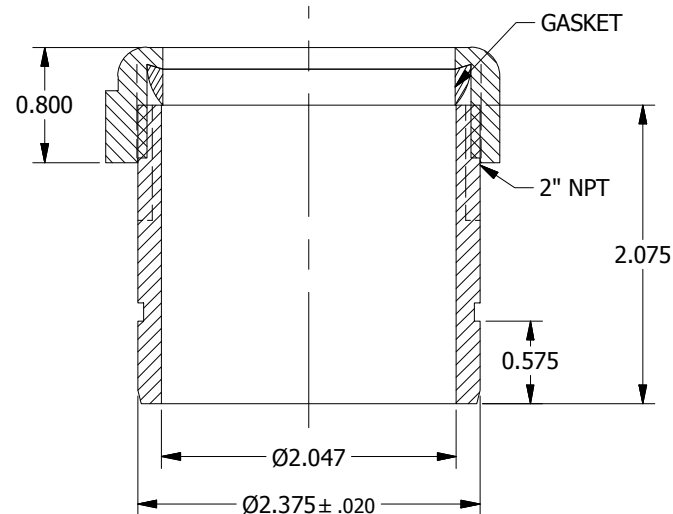
SECTION A-A
