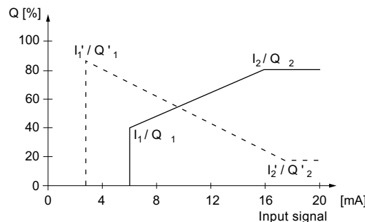
Fig. 10 Analog scaling
