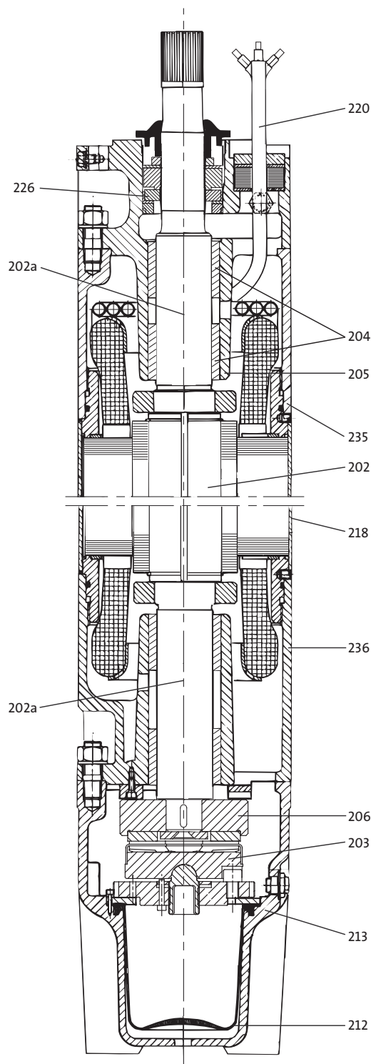
Fig. 20 MMS 10000
