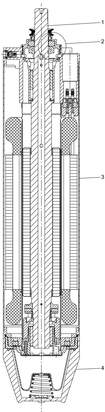
Fig. 19 MS6 motor
