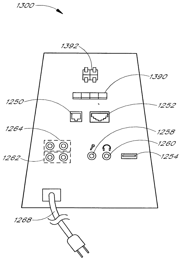
FIG. 13B
