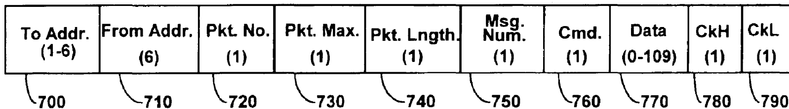
FIG. 7 Message Structure
