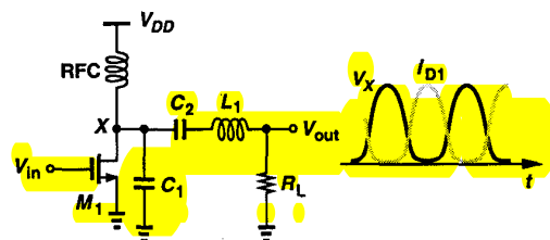
Fig. 29. Class E stage.
