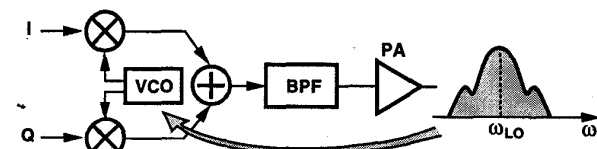
Fig. 17. LO pulling by PA.
