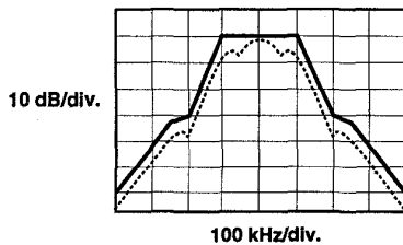
Fig. 13. GSM emission mask.
