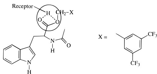
24 , L-732,138
