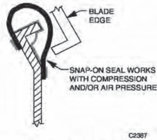
Fig. 5. Snap-On Blade Edge Seal.
