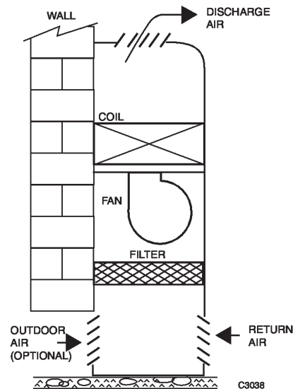
Fig. 30. Fan Coil Unit.
