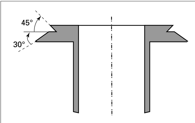
Fig. 24. Tapered flange.
