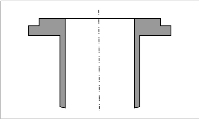
Fig. 23. Vertical flange.
