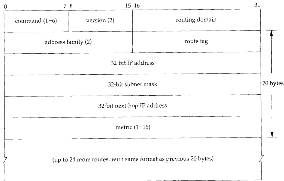
Figure 10.10 Format of a RIP-2 message.
