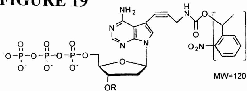
(Nitro-Benzyl)-dATP
