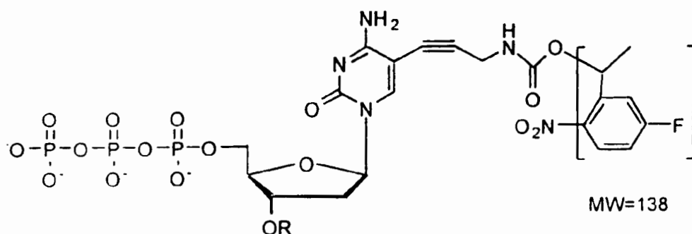
F-(Nitro-Benzyl)-dCTP
