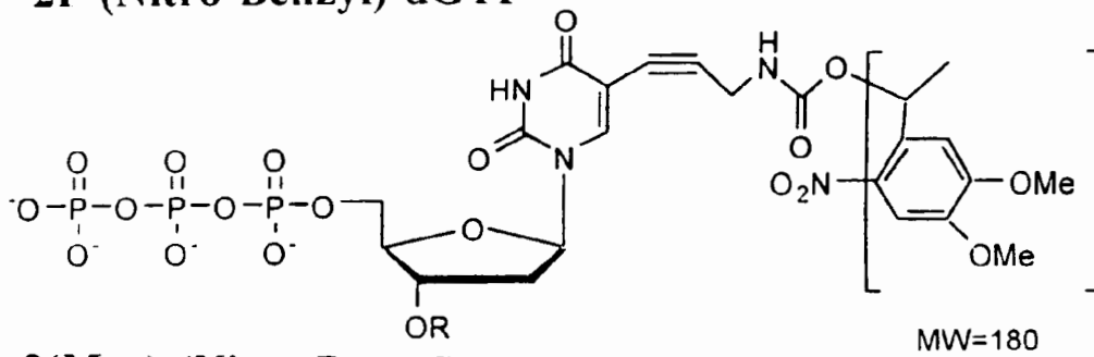
2(MeO)-(Nitro-Benzyl)-dTTP
