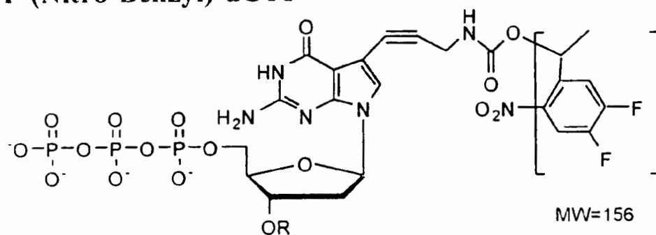
2F-(Nitro-Benzyl)-dGTP
