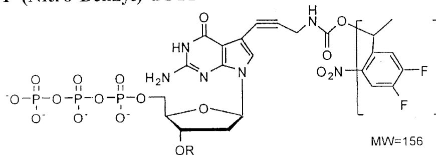
2F-(Nitro-Benzyl)-dGTP
