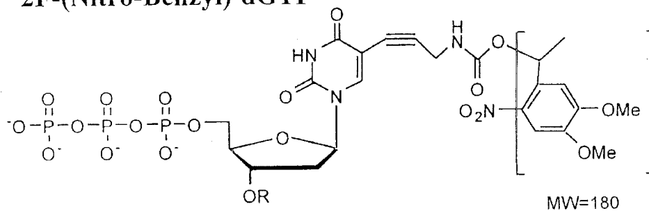
2(MeO)-(Nitro-Benzyl)-dTTP
