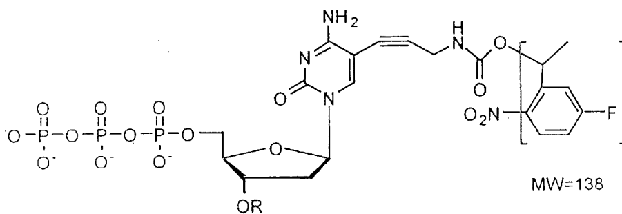
F-(Nitro-Benzyl)-dCTP
