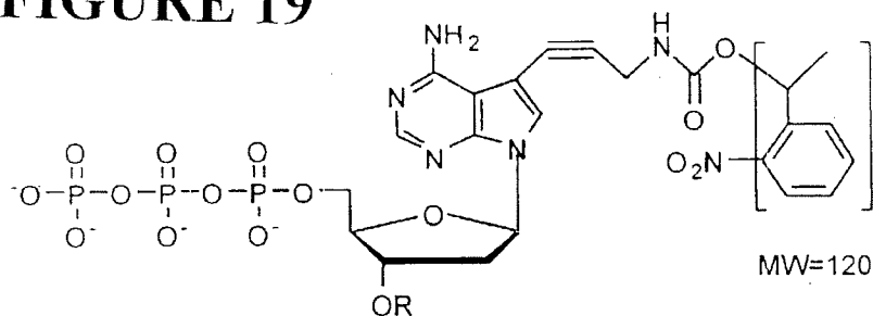
(Nitro-Benzyl)-dATP
