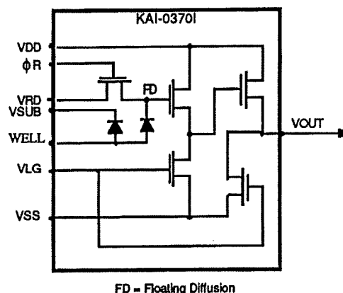
Fig. 5 CCD Output Schematic
