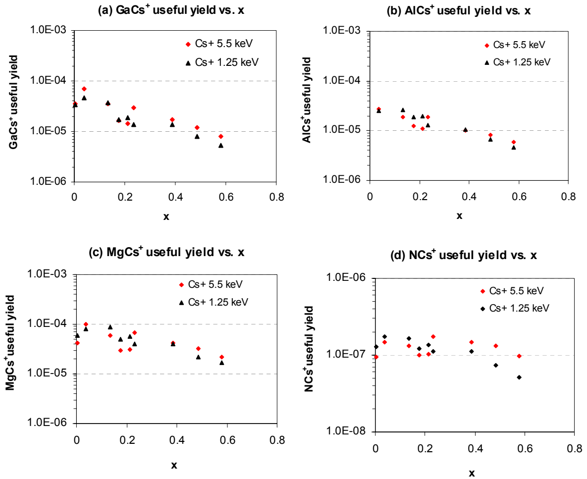
Figure 6-13. The useful ion yield of \text{MCs}^+ versus AlN mole fraction ( x ) in \text{Al}_x\text{Ga}_{1-x}\text{N} . (a) \text{GaCs}^+ ; (b) \text{AlCs}^+ ; (c) \text{MgCs}^+ and (d) \text{NCs}^+
