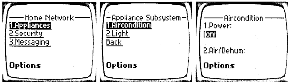
Fig. 9. HNS status.
