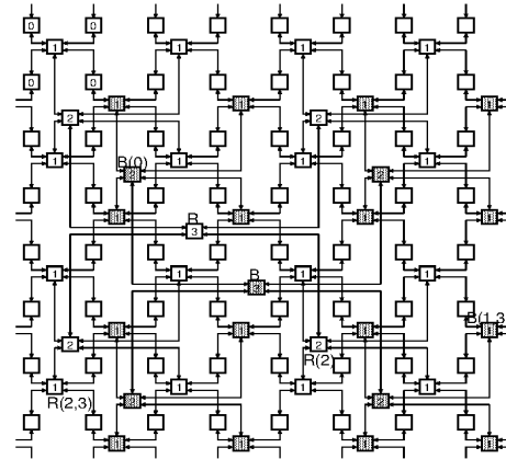
Fig. 4. Fat H-Tree
