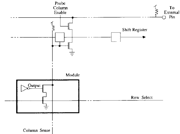
Fig. 7. Probe circuit.
