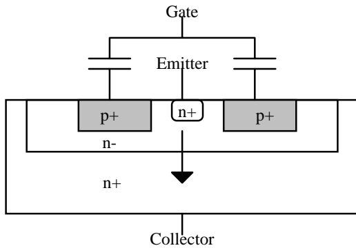
Fig. 9. Olympus SIT pixel.
