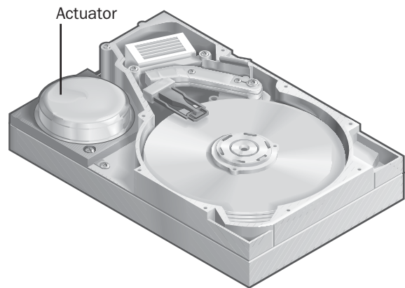
Actuator.
