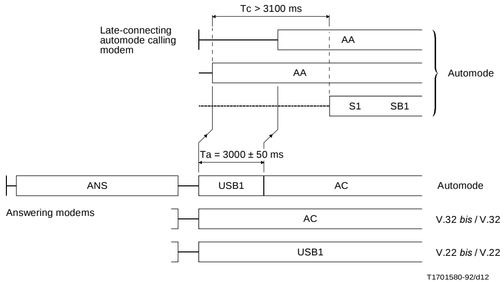
FIGURE A-3/V.32 bis
