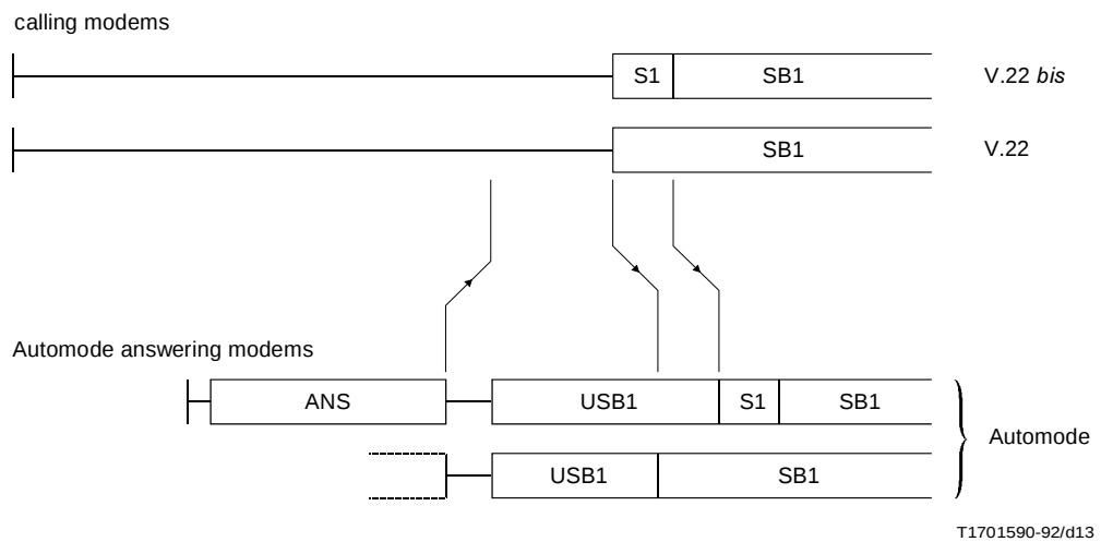
FIGURE A-4/V.32 bis
