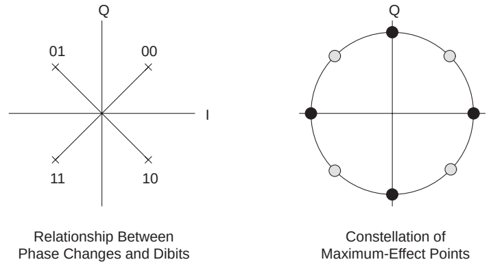
Figure 1. \pi/4 DQPSK
