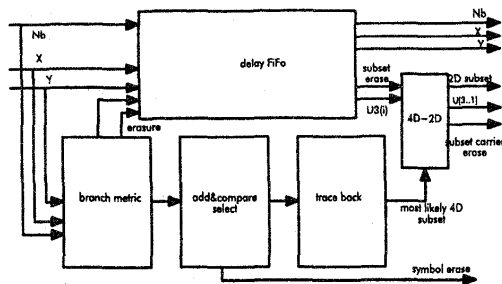
Fig. 6: Viterbi decoder.
