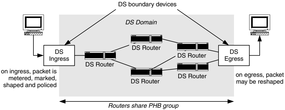
Figure 5.38 DS domain
