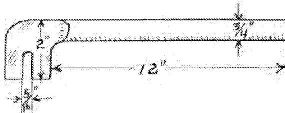
Timer Rod Bending Iron.
