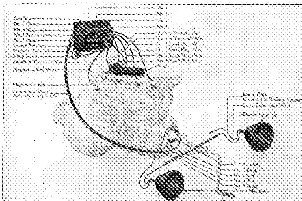
Wiring Diagram.
