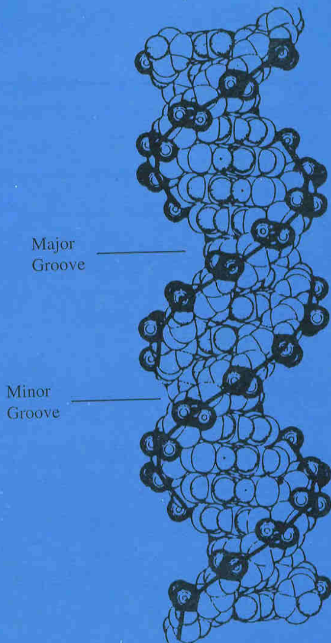
B-DNA
